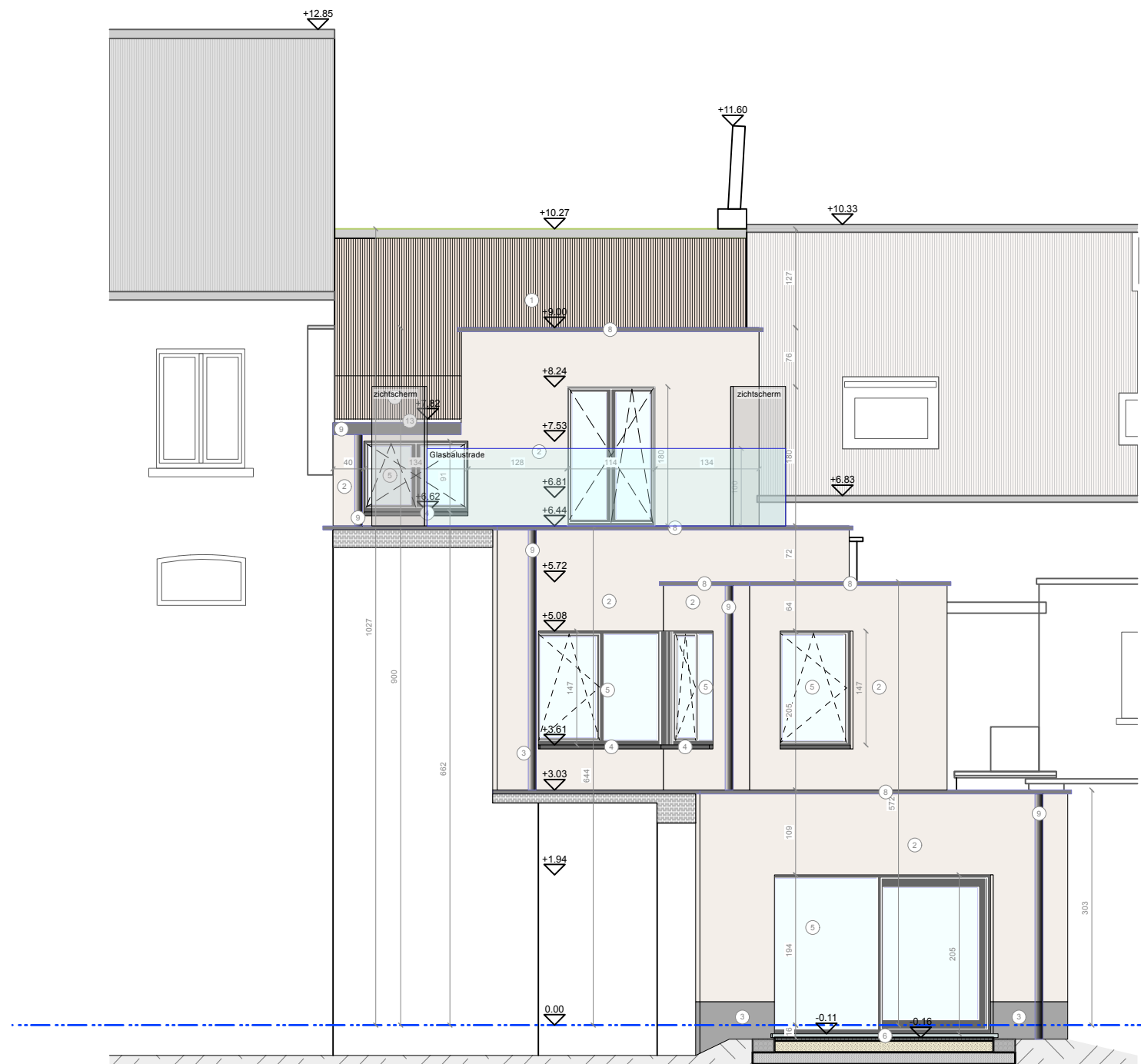
ACHTERGEVEL
